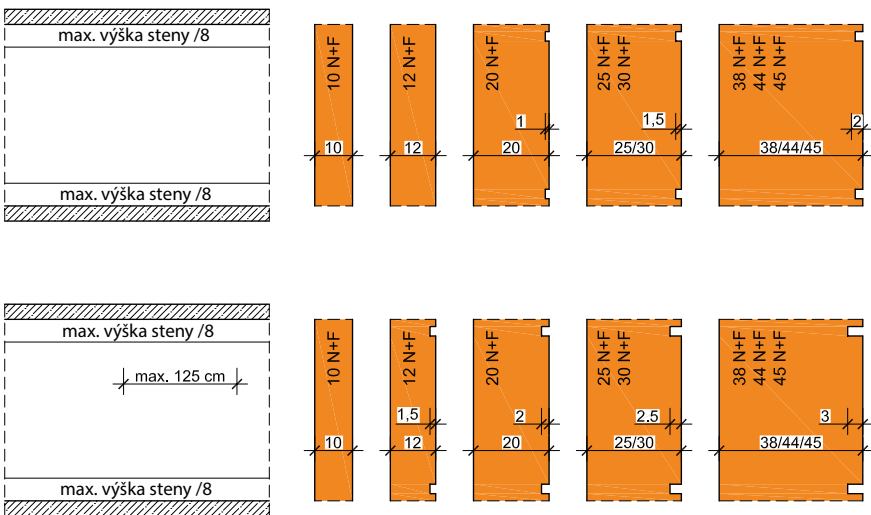
9. Najväčší rozmer vodorovnej drážky (ľubovoľná dĺžka drážky a pri dĺžke max. 125 mm).
