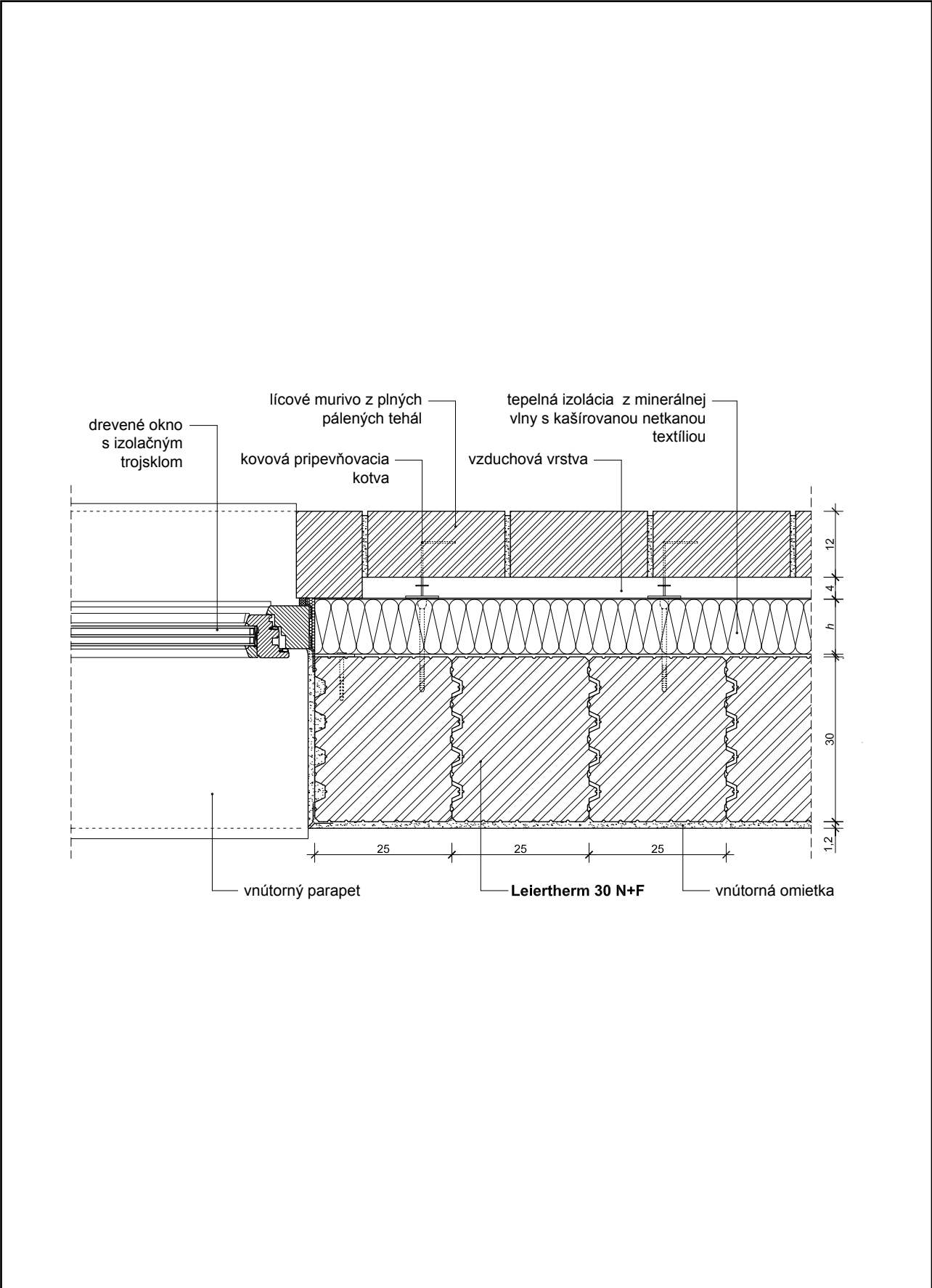
31/32 Zabudovanie okien – odvetraná fasáda vodorovný rez Leiertherm 30 N+F 1:10
