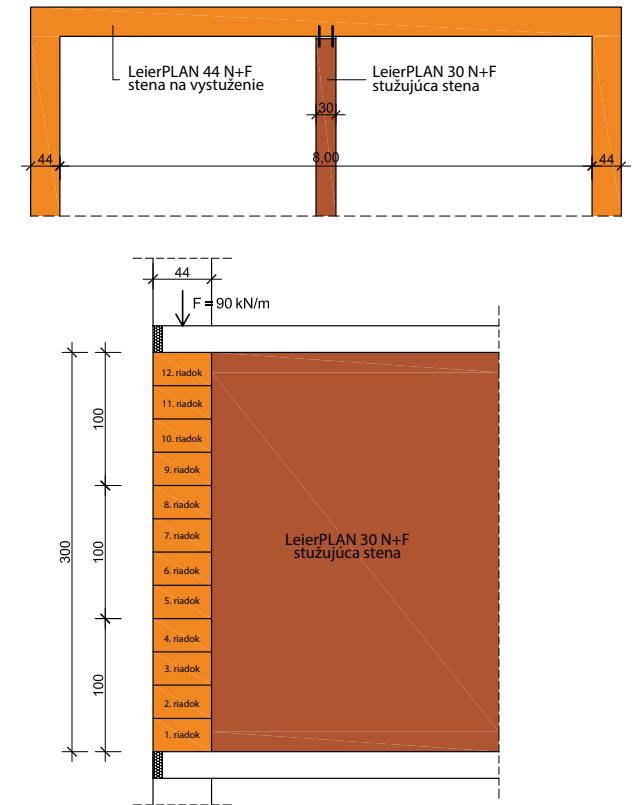
5. Výpočet stenovej spony
