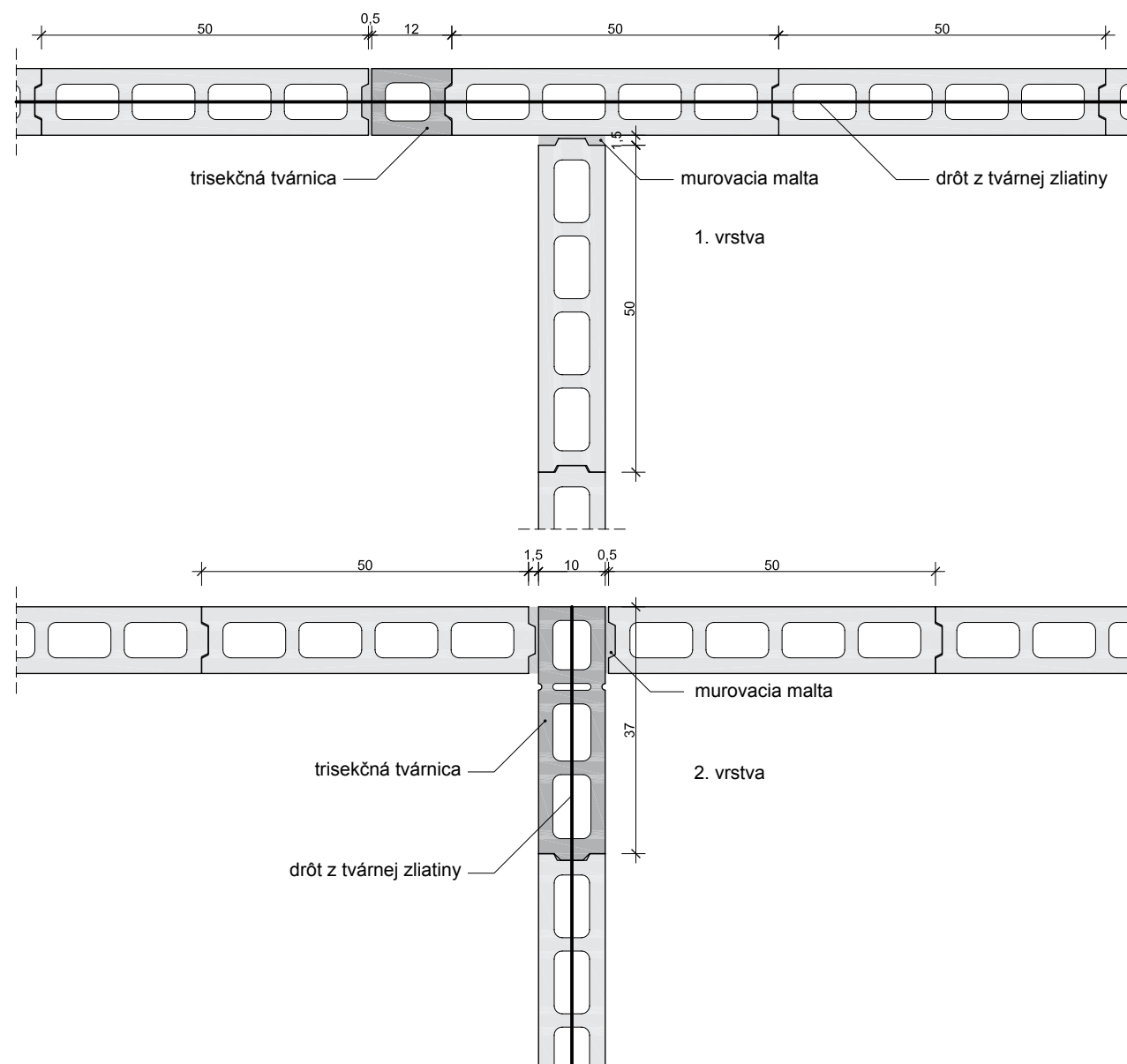
25. Roh steny: Betónová priečkovka Leier VF10
