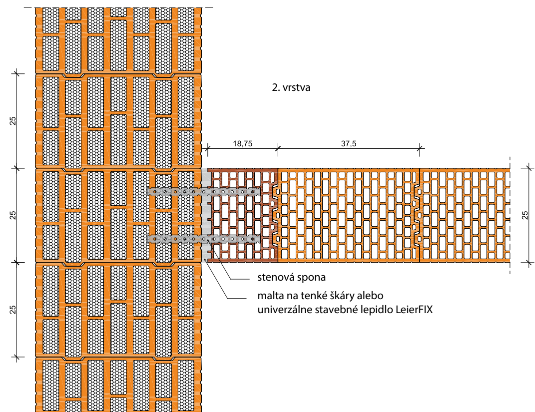
76. Pripojenie steny: LeierPLAN 44 ISO+ – LeierPLAN 25 N+F
