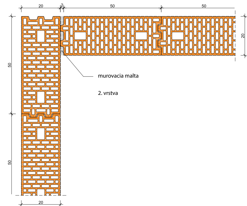
59. Roh steny: Leiertherm 20 N+F
