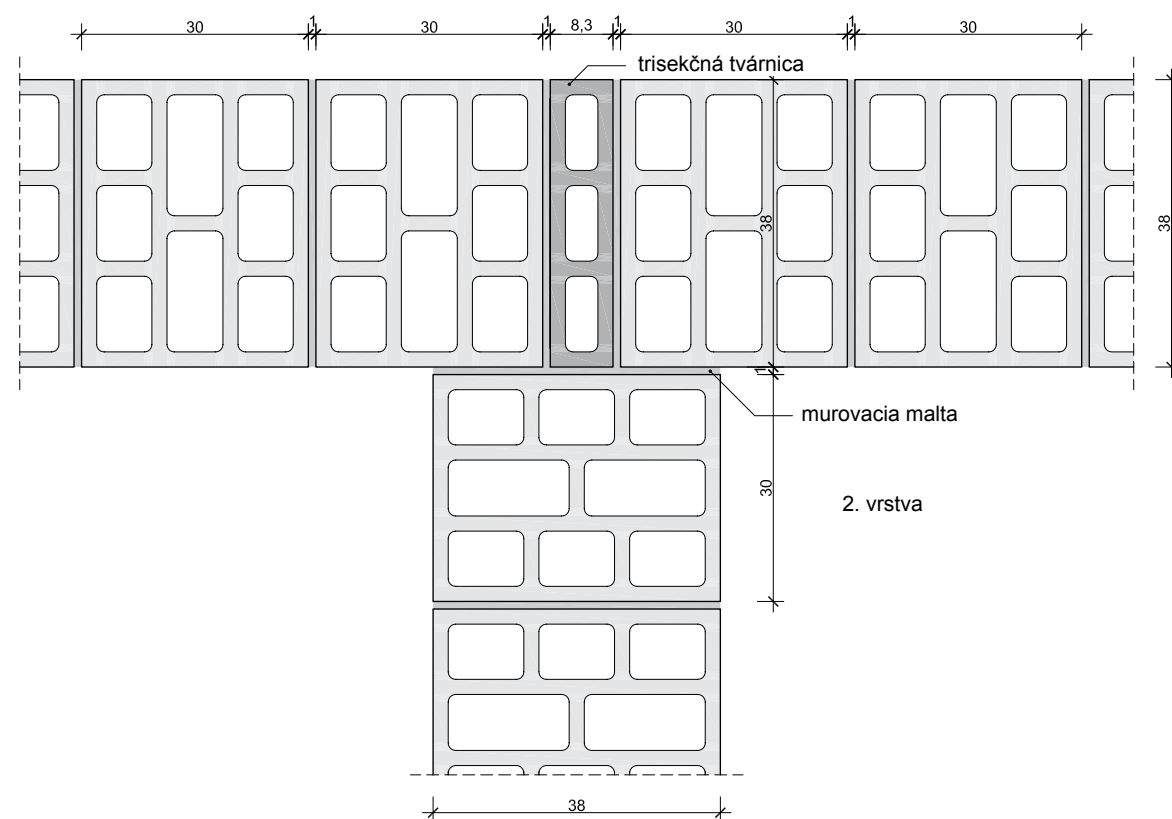
14. Prípojenie steny: Leier – pívničná murovacia tvárnica UNI (38cm)
