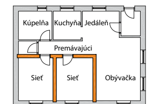
29. Steny oddelujúce tiché a hlučné zóny
