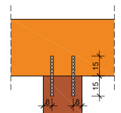
19. Bekötőszalag helye
