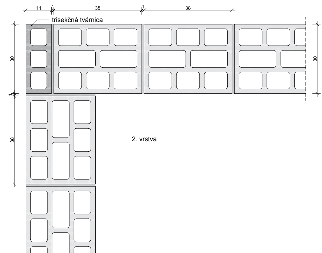
15. Roh steny: Leier – pívničná murovacia tvárnica UNI (30cm)
