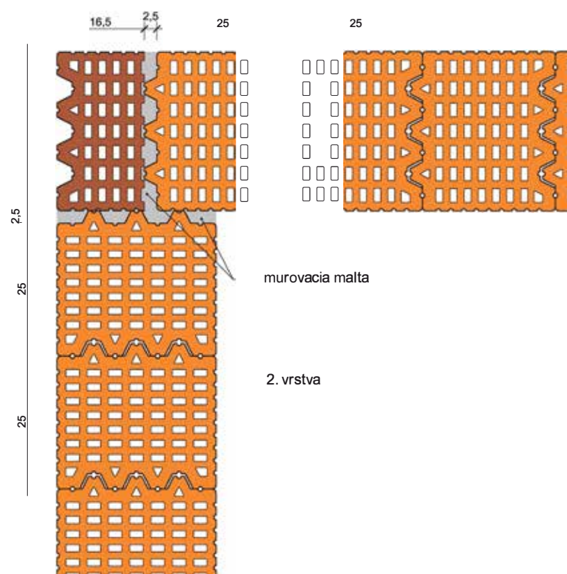
88. Vázba rohu steny Leiertherm 30 N+F AKU
