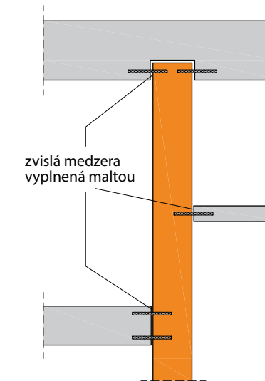
31. Použitie stenovej spony
