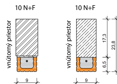
18. Možnosti uloženia prekladu Leier MDA
