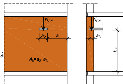
3. Výklad záťaženej plochy pri koncentrovanej sile
