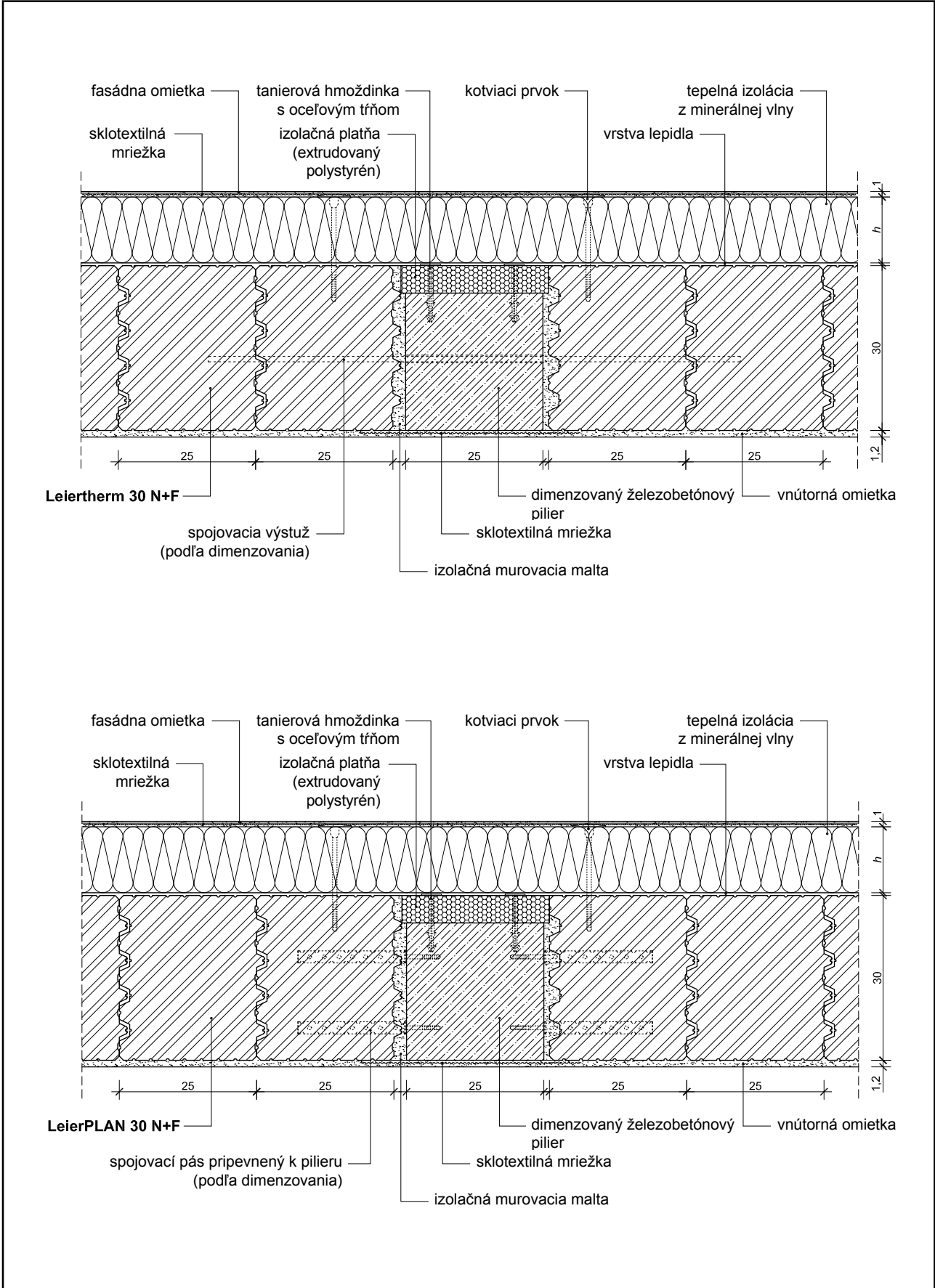
32/32 Výplňová stena – železobetónový pilier vodorovný rez Leiertherm 30 N+F LeierPLAN 30 N+F 1:10
