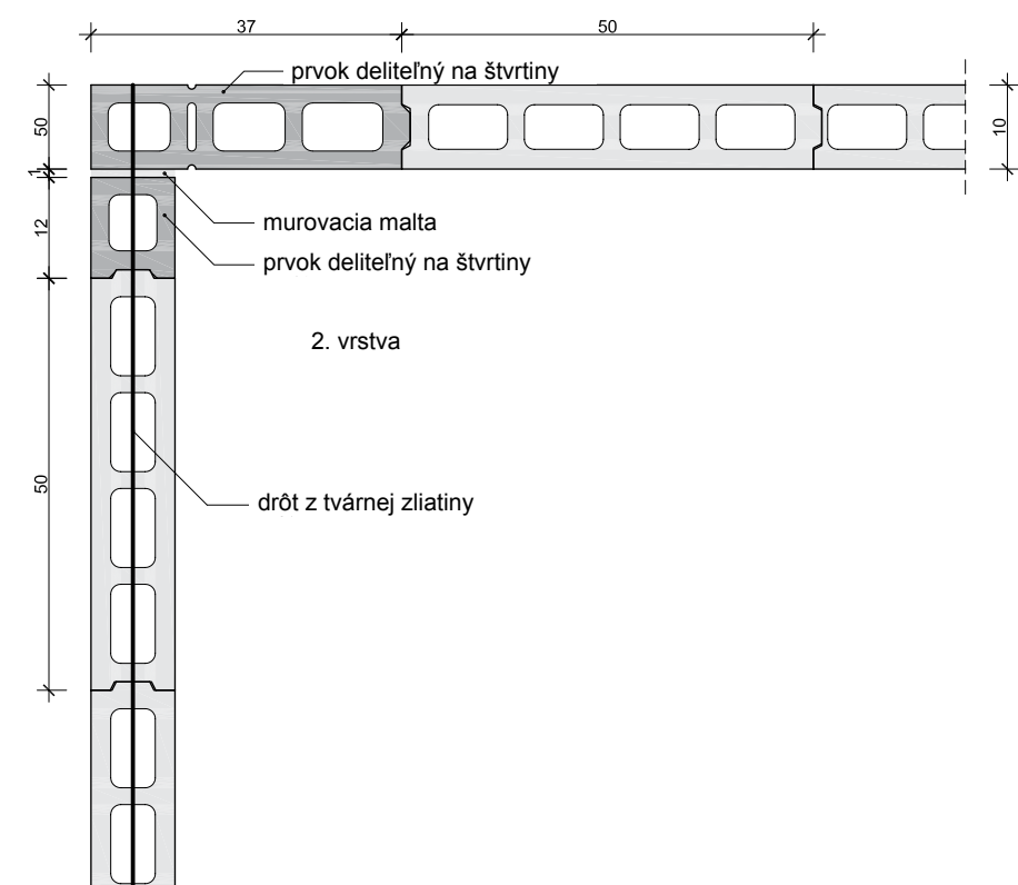
23. Roh steny: Betónová priečkovka Leier VF10
