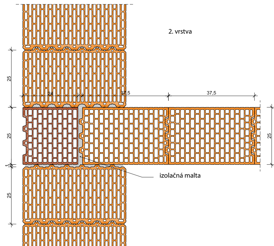
74. Pripojenie steny: Leiertherm 45 N+F – Leiertherm 25 N+F
