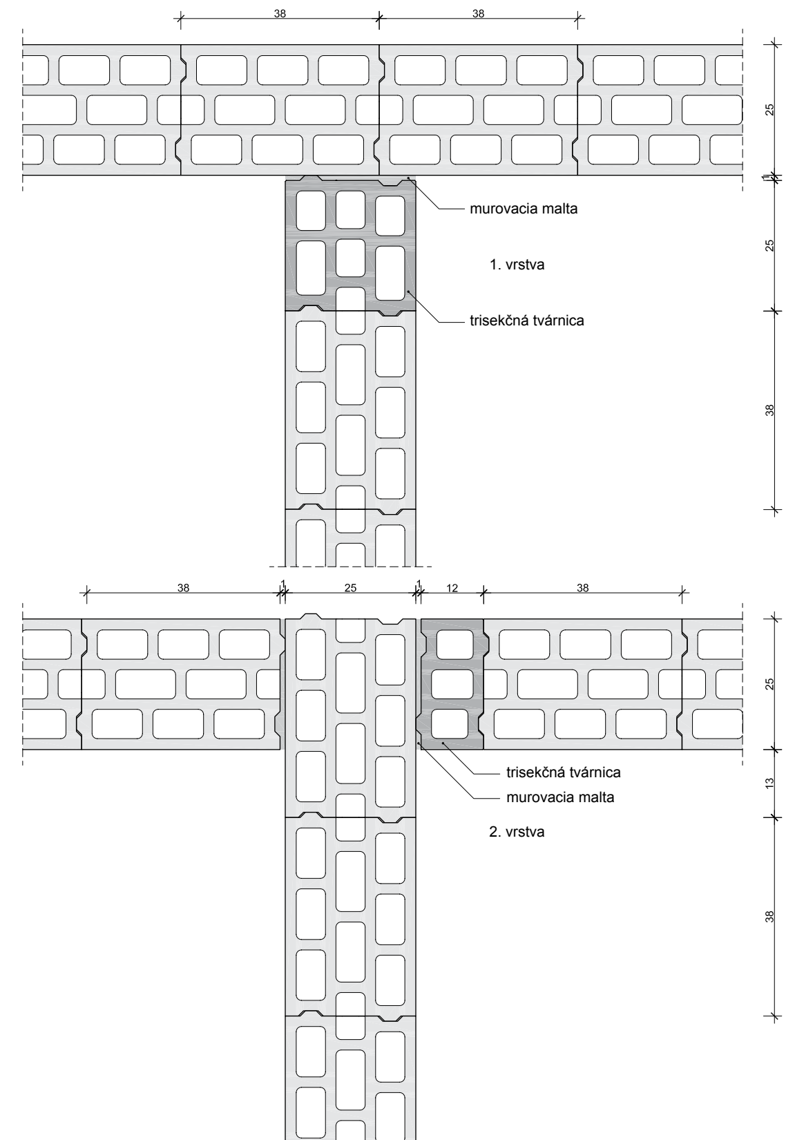
19. Pripojenie steny: Betónová murovací tvárnica Leier FF 25
