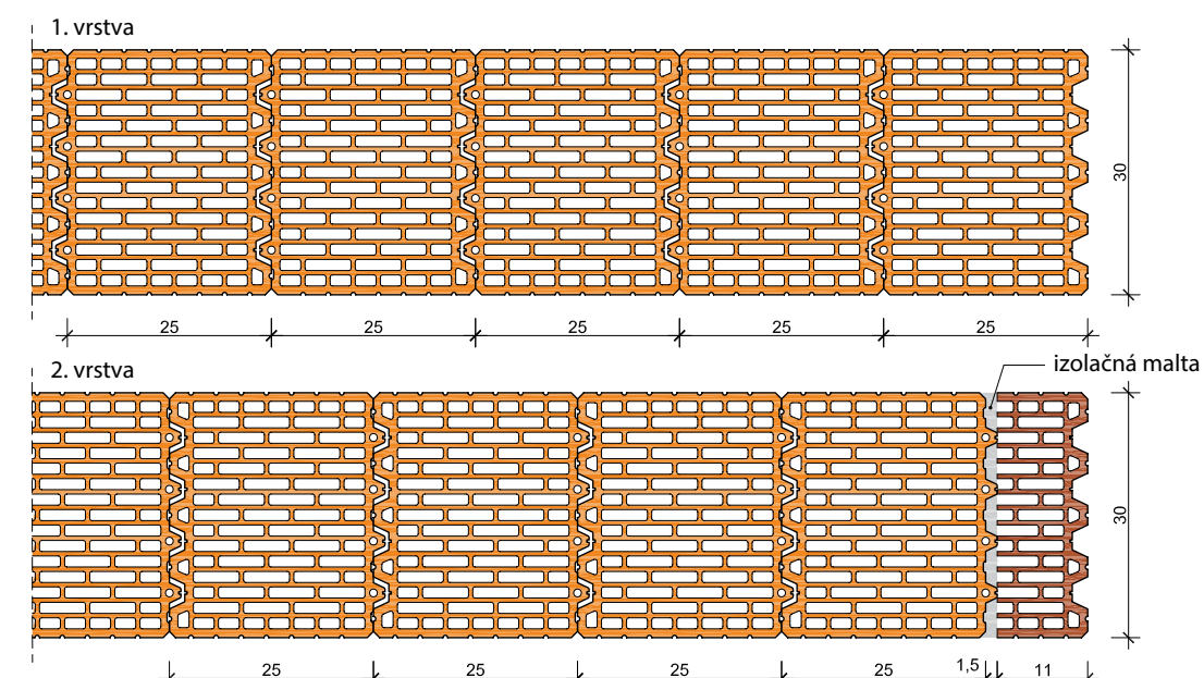
55. Koniec steny: Leiertherm 30 N+F alebo LeierPLAN 30 N+F
