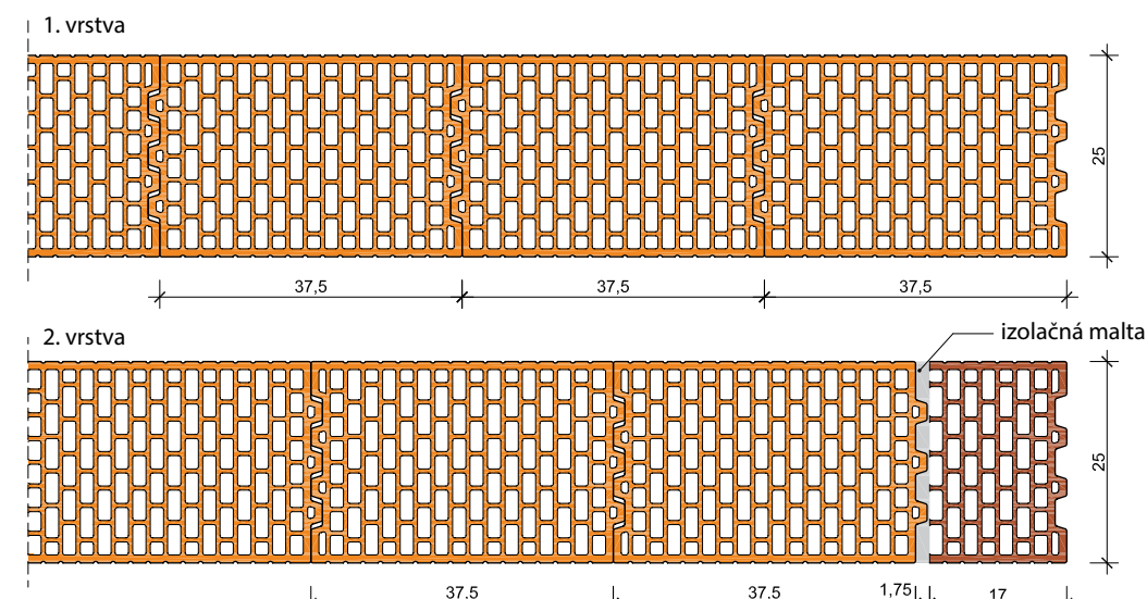
54. Koniec steny: Leiertherm 25 N+F alebo LeierPLAN 25 N+F
