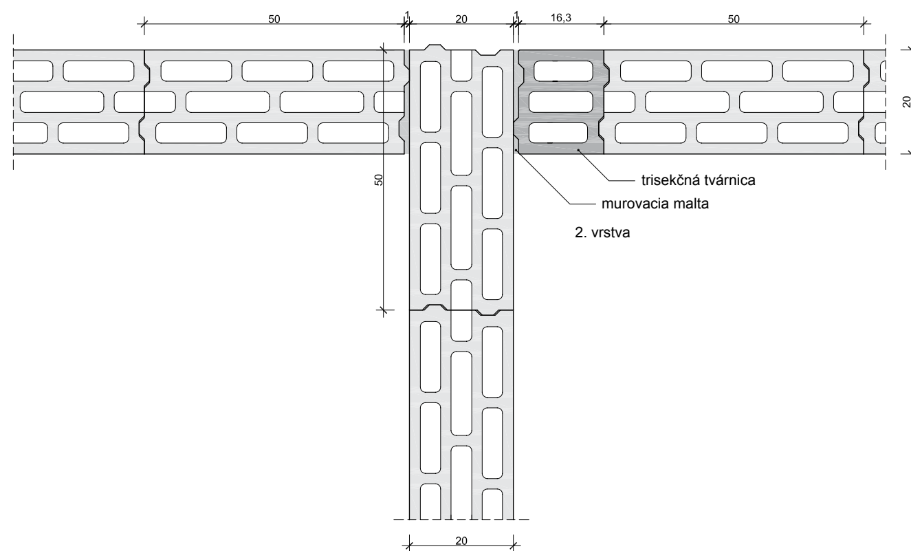
22. Pripojenie steny: Betónová murovacia tvárnica Leier FF 20
