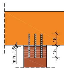
3. Umiestnenie jednej, dvoch a troch stenových spôn
