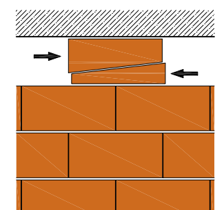
5. Rezanie tvárnice
