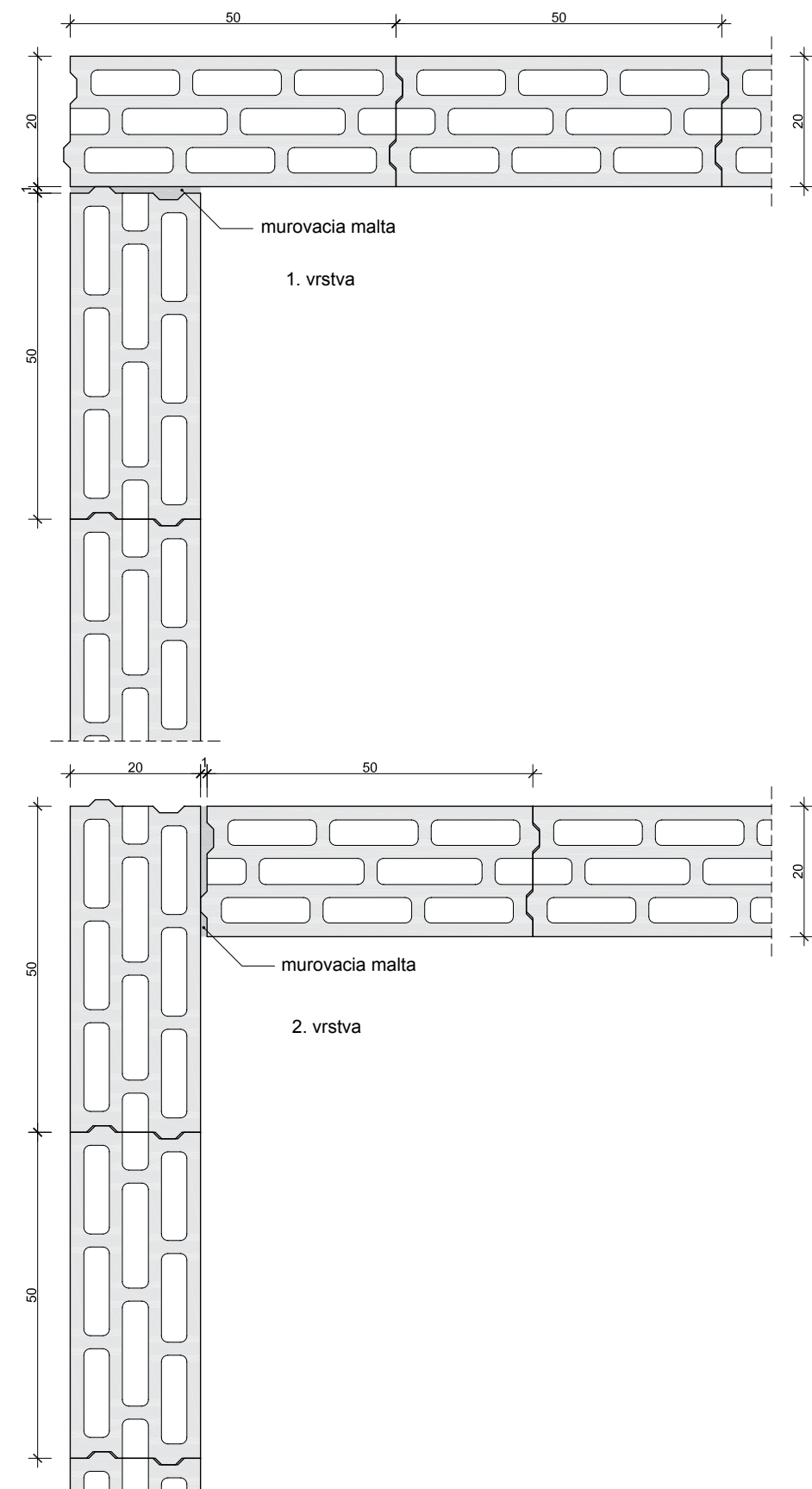
21. Roh steny: Betónová murovacia tvárnica Leier FF 20
