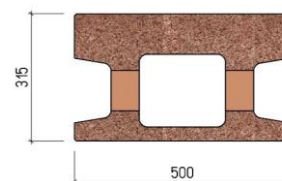
N - tvarovka (normál - priebežná)
