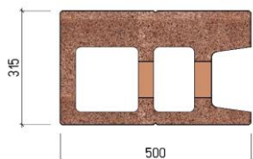
U - tvarovka (univerzálna)
